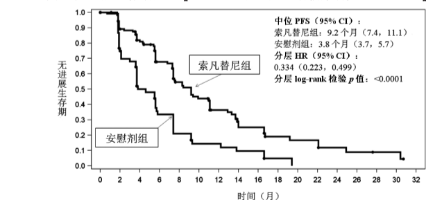
图1 无进展生存期的Kaplan-Meier曲线-III期临床研究（SANET-ep）
