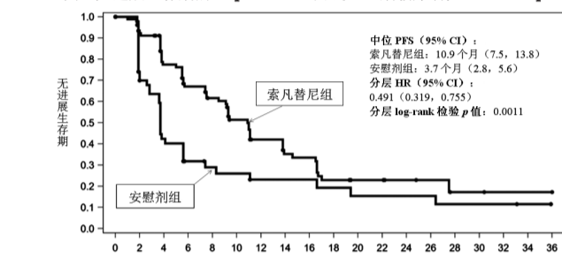
图2 无进展生存期的Kaplan-Meier曲线-III期临床研究（SANET-p）
